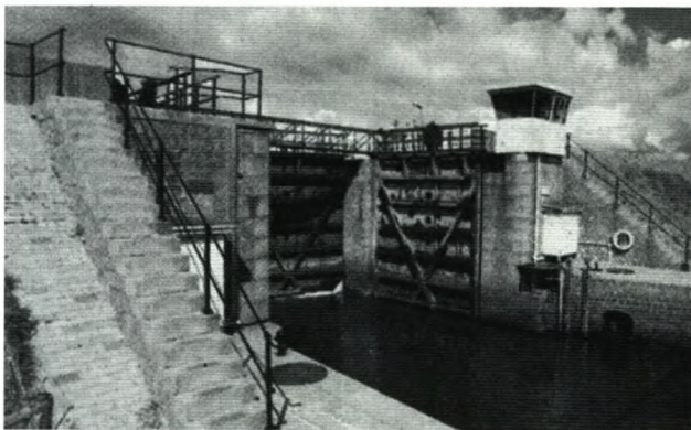
Kammerslusen er et logisk navn til slusen, da skibene sejler ind i en sluse, hvor vandstanden så hæves eller sænkes til niveauet i Vadehavet ved højvande. Er der lavvandet, passer vandstanden, og så er portene åbne.
